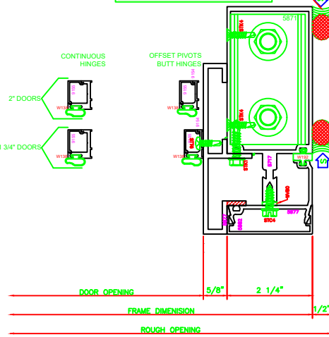
8164 O.G. JAMB 5600 6"
