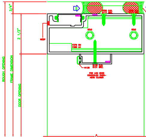
8162 HEADER 5600 6"
